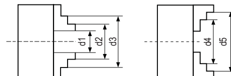
Spannbereich Dreibacken-Drehfutter
