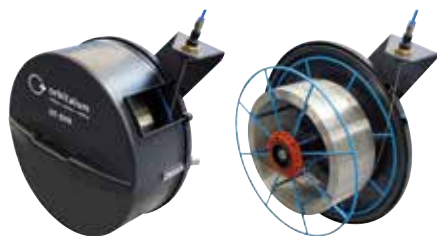
Kaltdrahtzuführung DVR 100 (mit und ohne Abdeckhaube)
