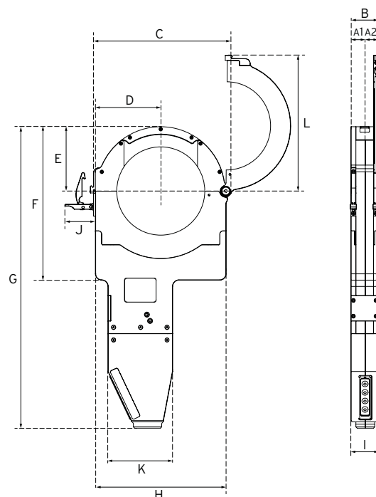
T-Stück-Spanneinsätze mit Aufnahmefähigkeit des ausgehalsten und des anzuschweißenden Rohres
